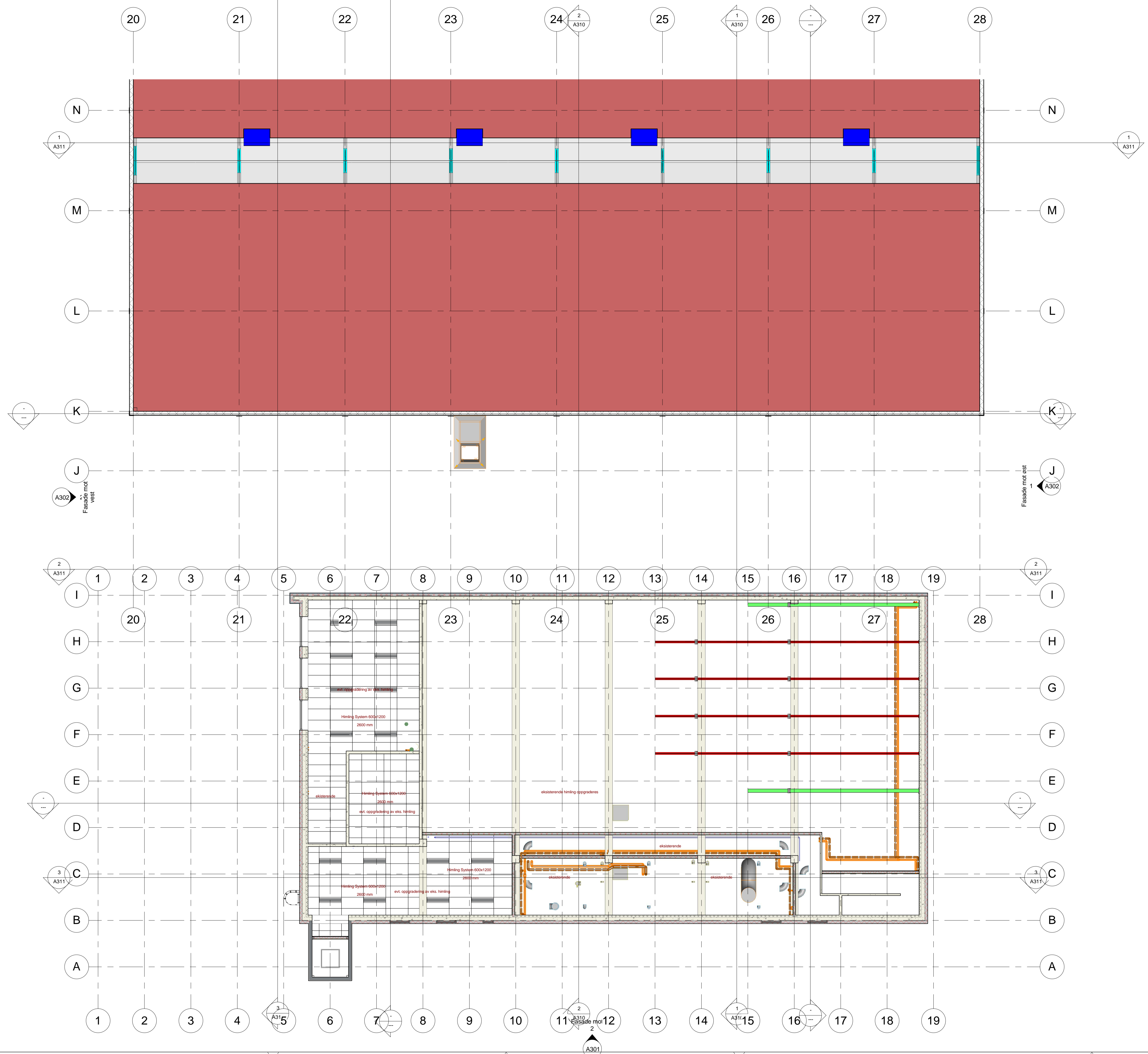
1 Plan 3 1 : 100
