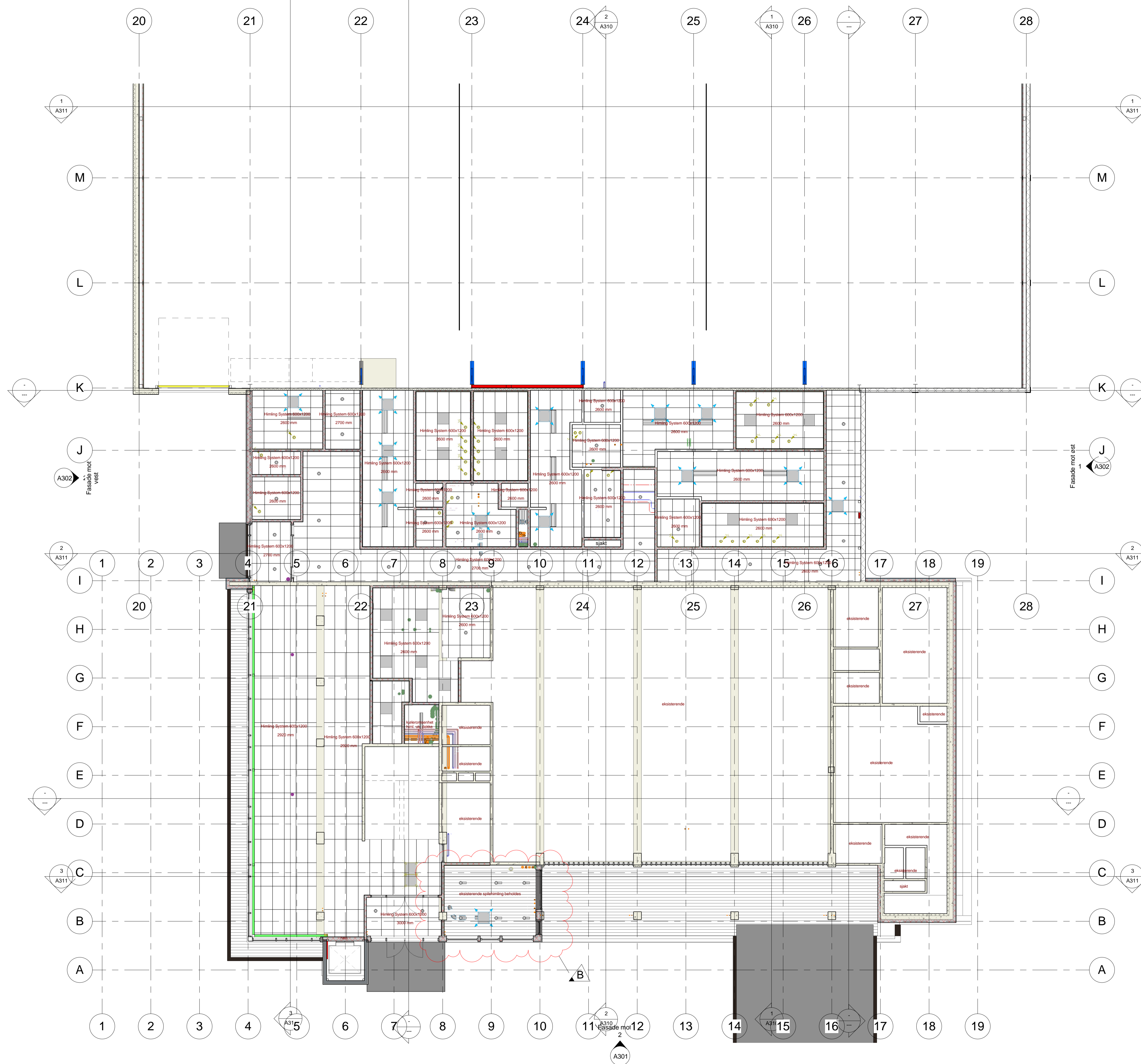
1 Plan 1 1:100
